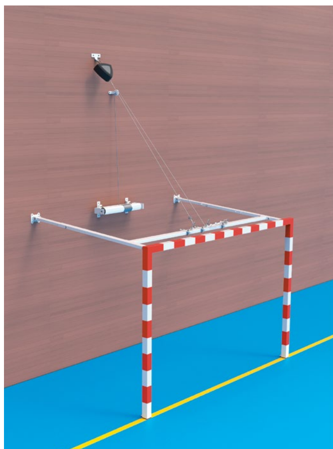
En fixation poteaux Réf. HB01N001
